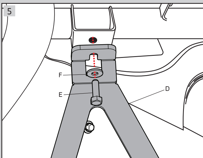
Connect rear bracket (D) using kit M8 (8.8) bolt Tightening torque 40Nm
